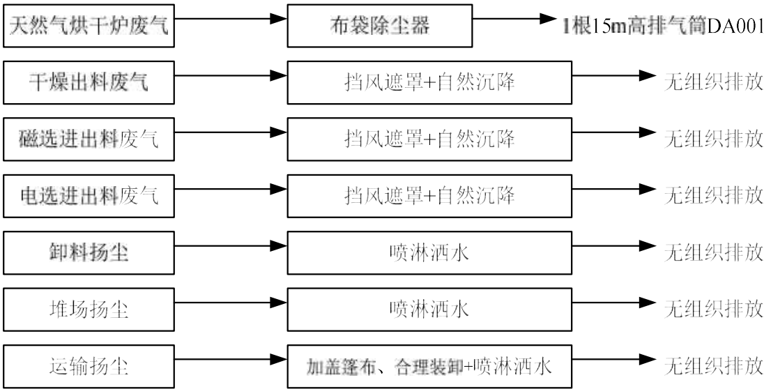
图 6.1-2 项目废气处理工艺流程图
